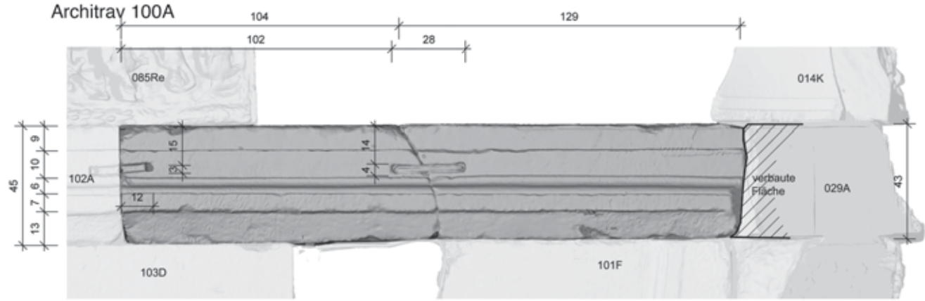
Ansicht Ost
