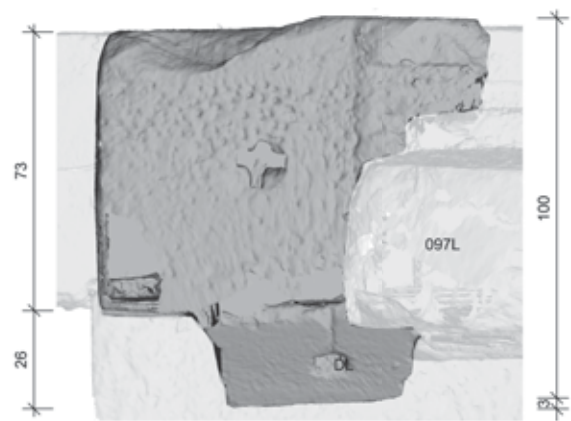
Draufsicht
