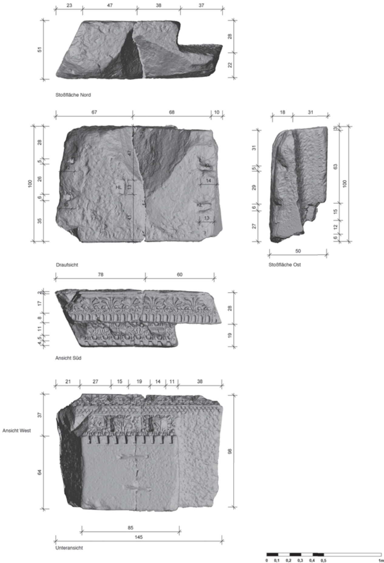
Schräggeison 054G
