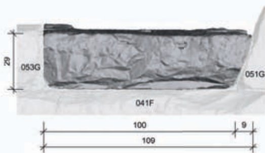
Stoßfläche Nord
