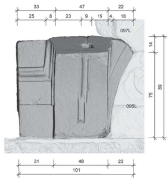
Ansicht Süd
