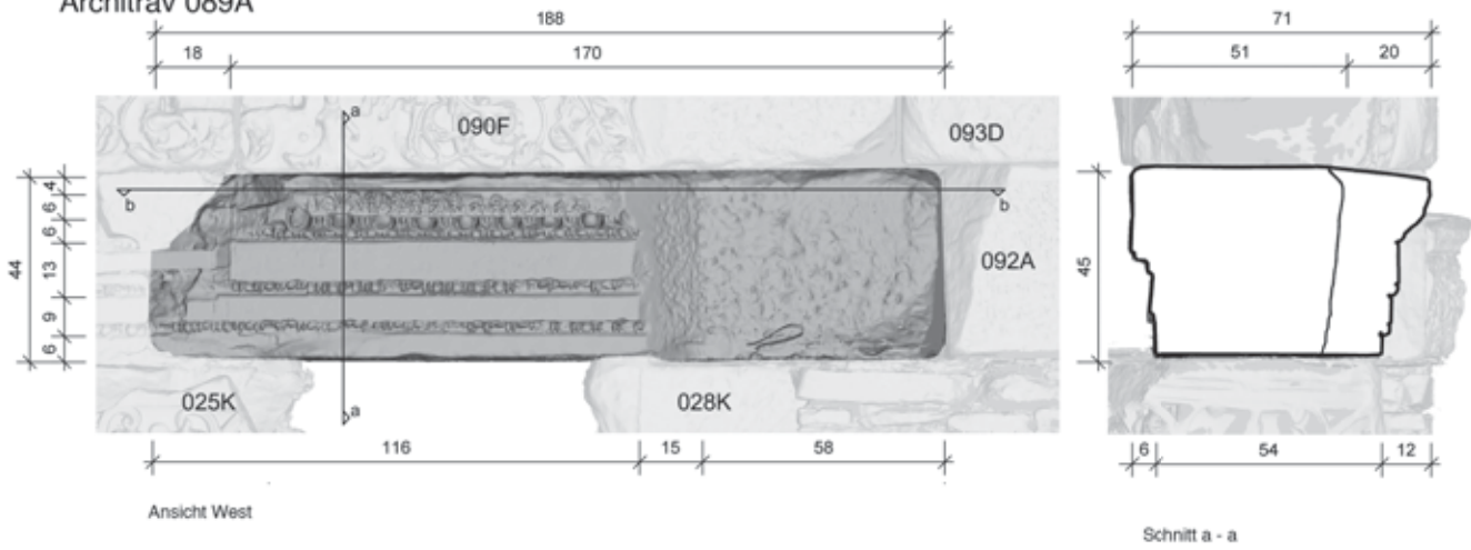
Architrav 089A
