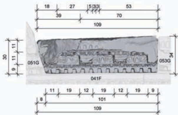
Ansicht Süd
