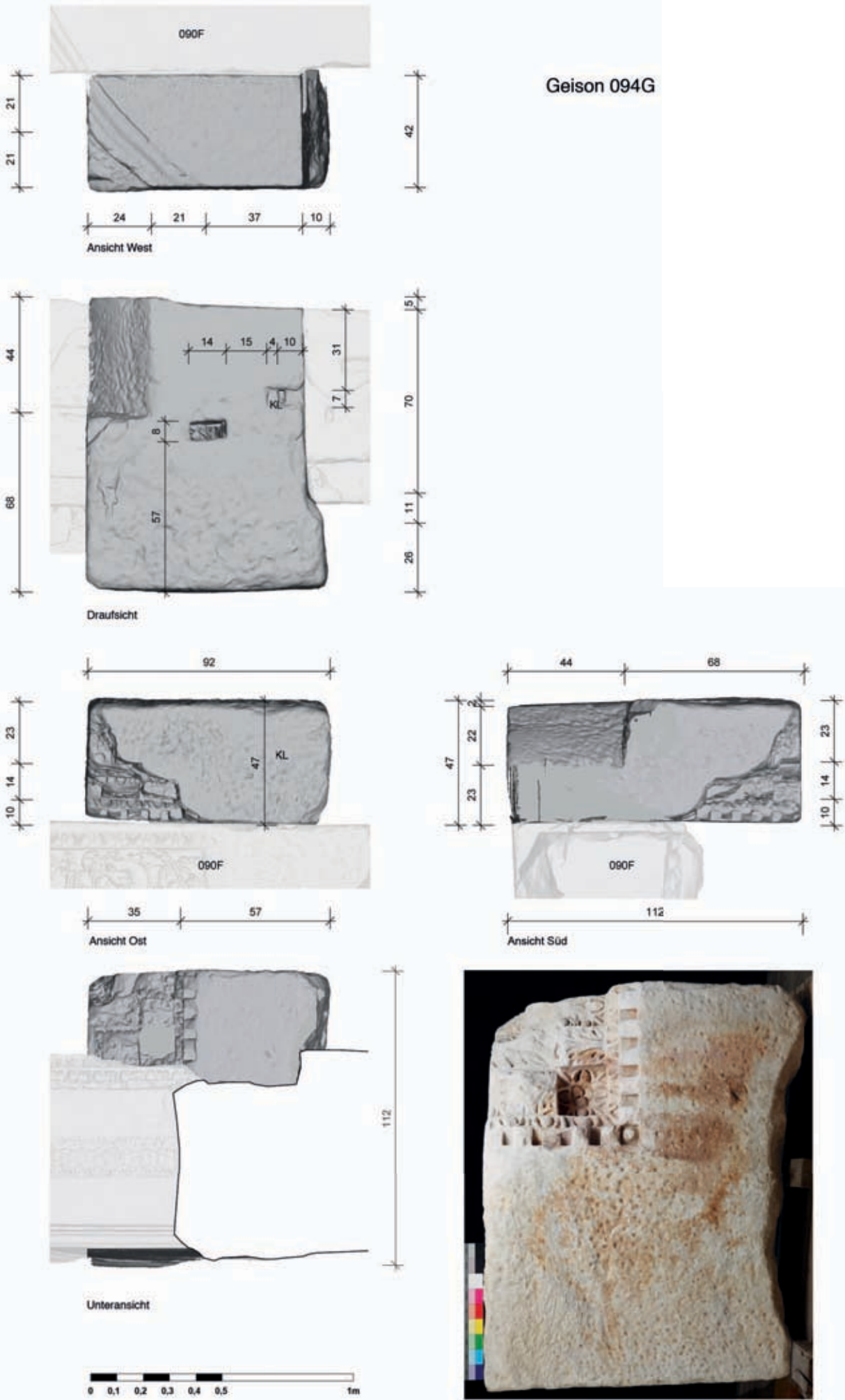
Geison 094G
