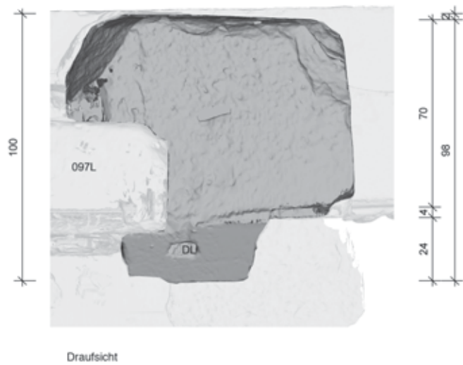
Draufsicht
