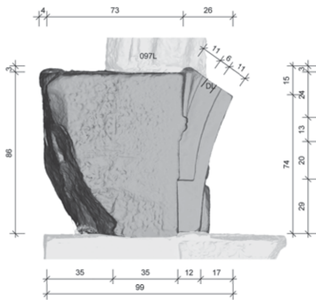
Ansicht West
